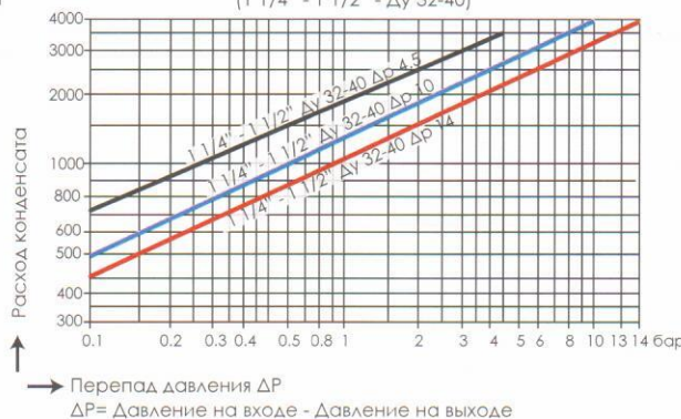
(1 1/4" - 1 1/2" - Ду 32-40)
