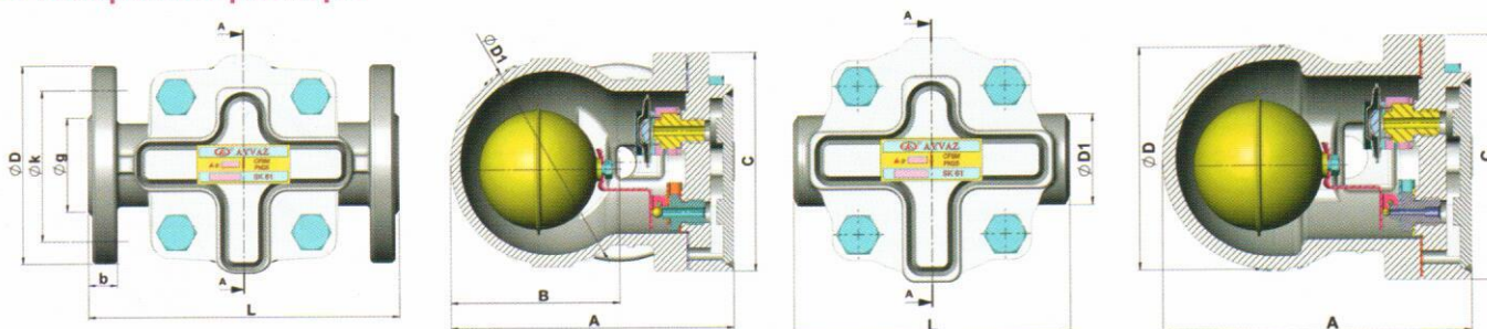
Габаритные размеры
